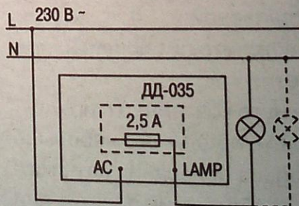
Рисунок 10. Схема подключения ДД-035
