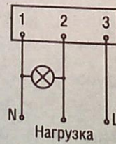
Рисунок 4. Наибольшая чувствительность
