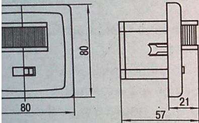
Рисунок 3. ДД-035
