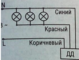
Рисунок 6. Схема подключения ДД-028
